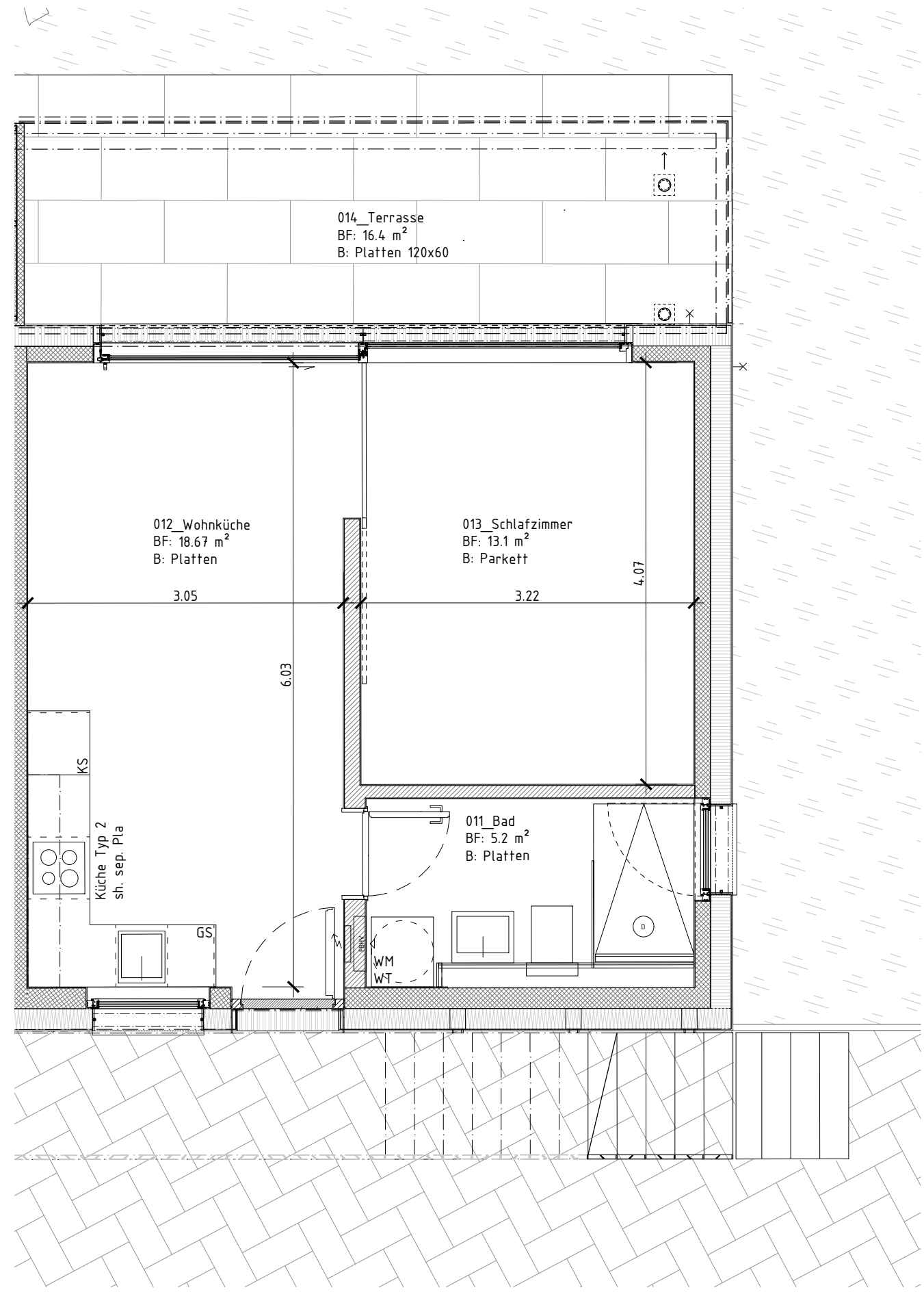
Haus 2 - Erdgeschoss Wohnung 2
