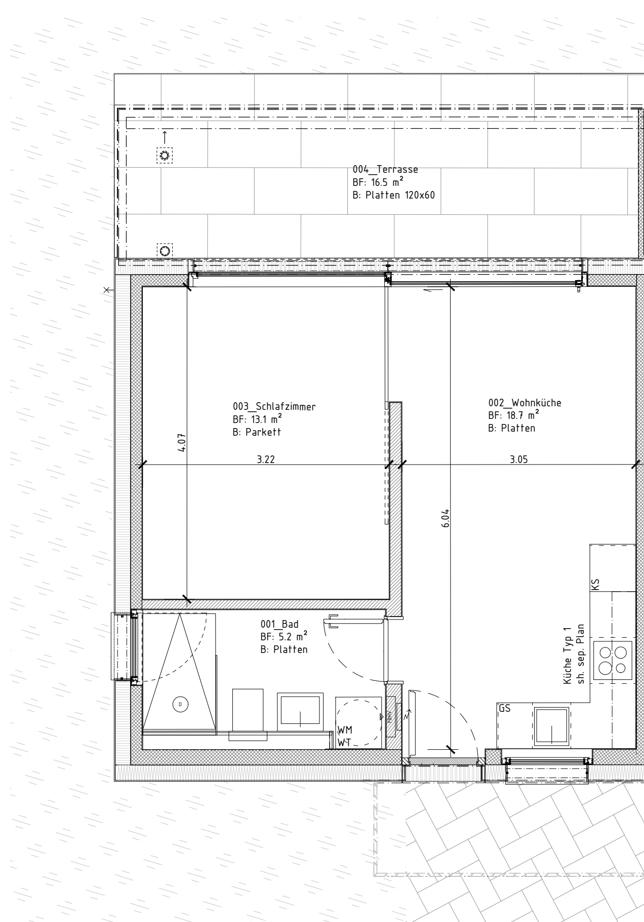
Haus 2 - Erdgeschoss Wohnung 1
