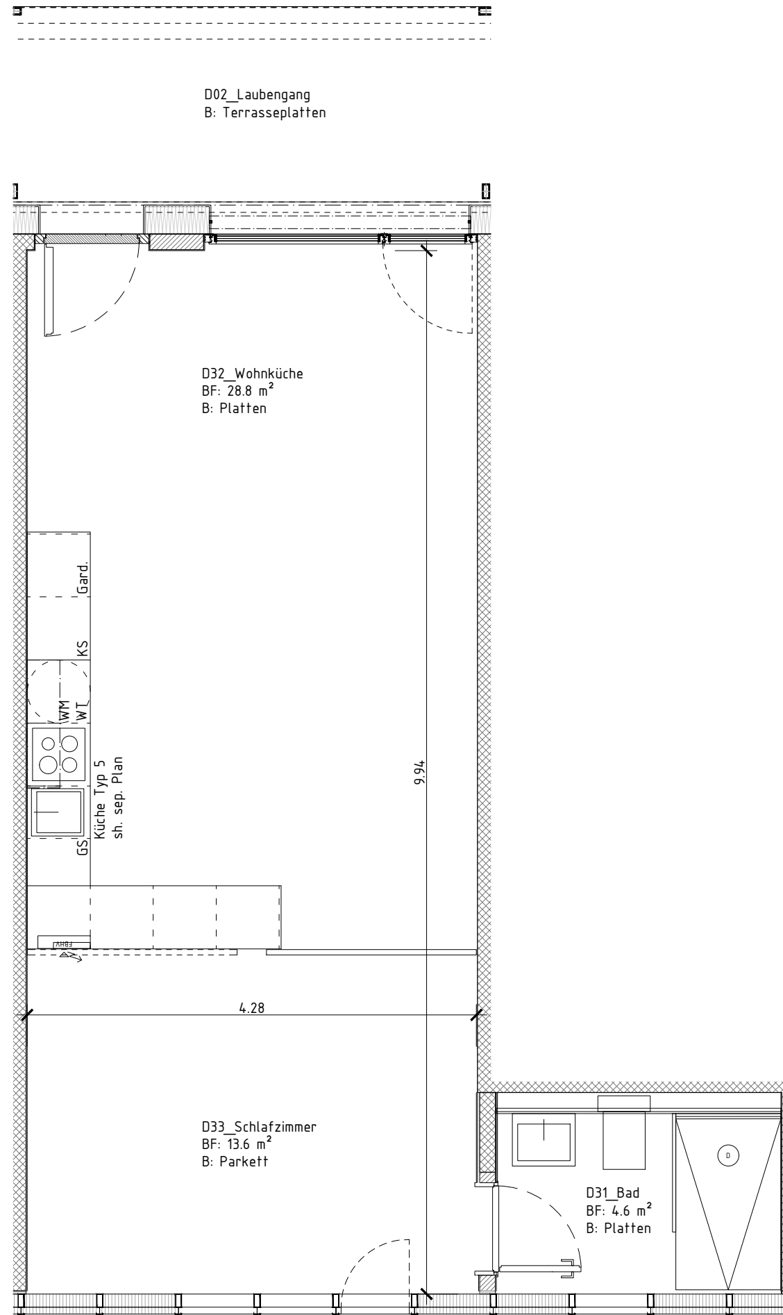
Haus 1 - 2.Obergeschoss Wohnung 8
