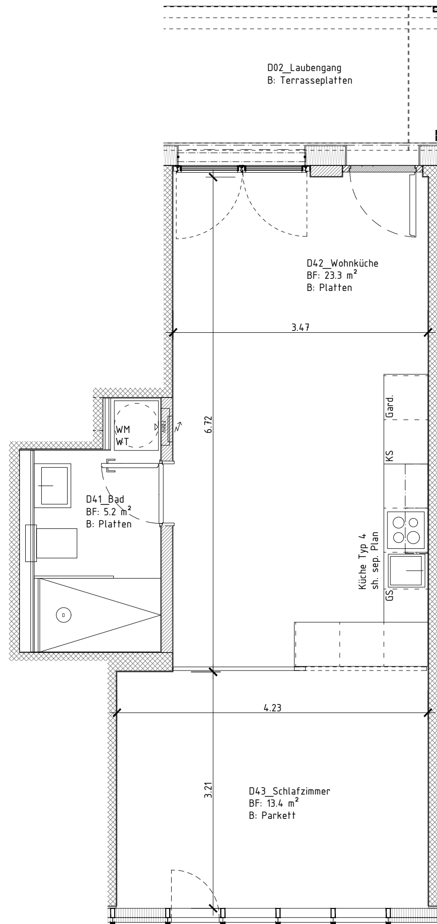
Haus 1 - 2.Obergeschoss Wohnung 7
