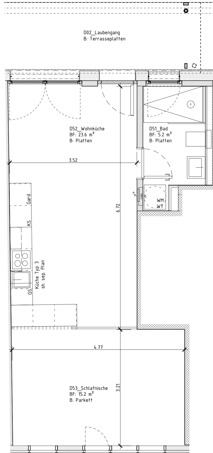
Haus 1 - 1.Obergeschoss Wohnung 1
